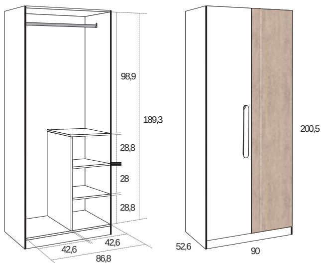
ARMÁRIO 2 PORTAS 90cm. (201)
