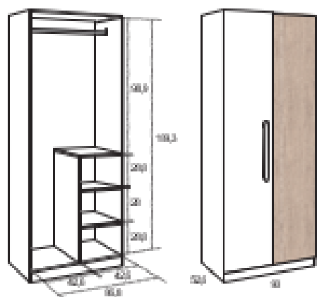
ARMÁRIO 2 PORTAS 90cm. (201)
